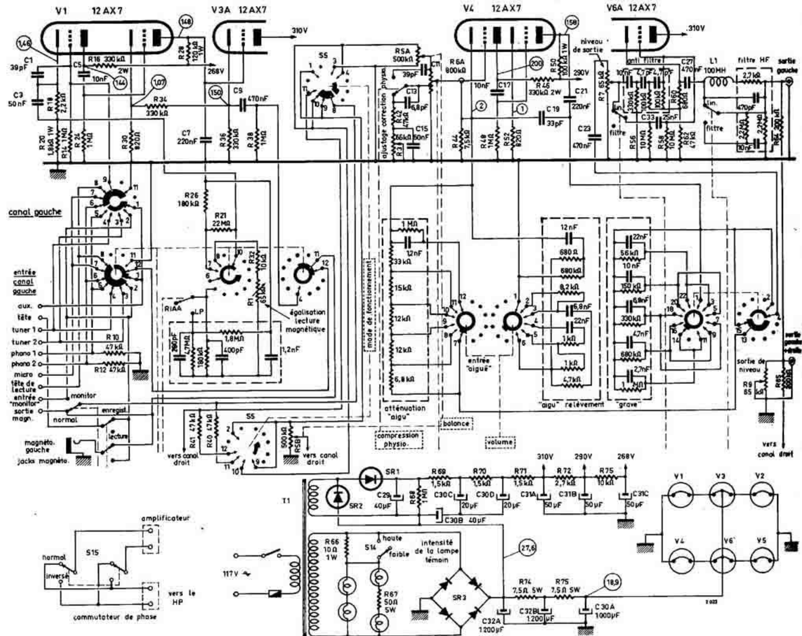
Schéma du préamplificateur McIntosh C 22. On a représenté ici l'un des deux canaux.
