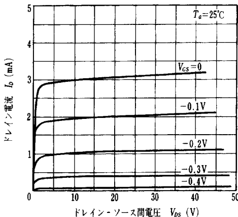
I_D - V_{DS} 特性
