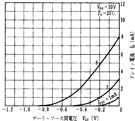
I_D - V_{GS} 特性
