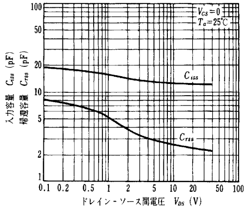
C_{iss}, C_{rss} - V_{DS} 特性
