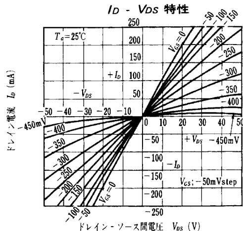
I_D - V_{DS} 特性
