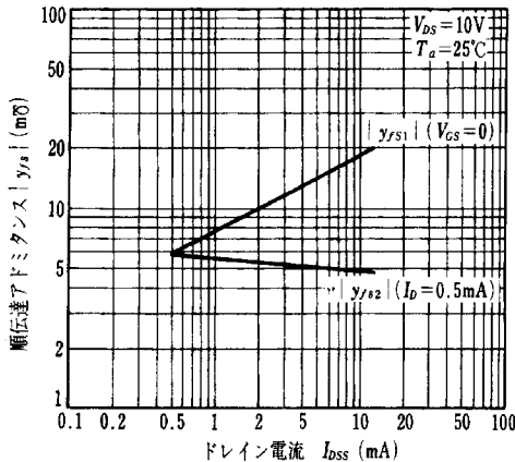
|y_{fs}| - I_{DSS} 相関図
